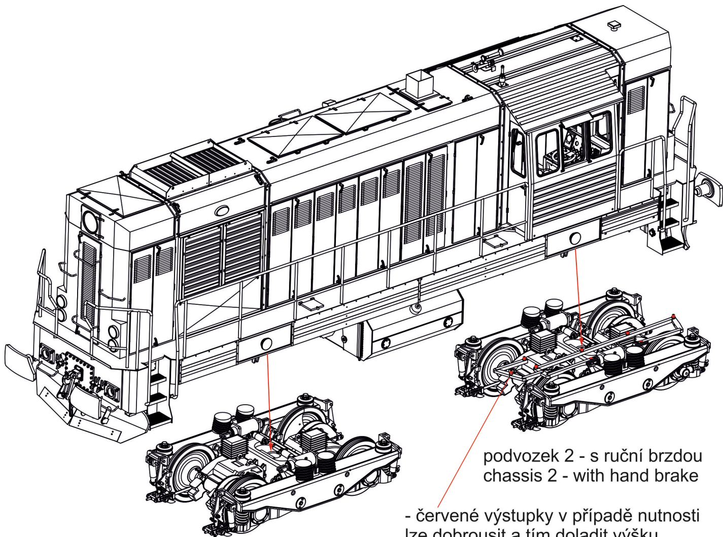
podvozek 1 - bez ruční brzdy chassis 1 - without hand brake
